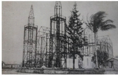
Estructura metálica del Templo Parroquial de San Ramón. Cerca de 1930. Colección Museo Regional de San Ramón, Universidad de Costa Rica.
